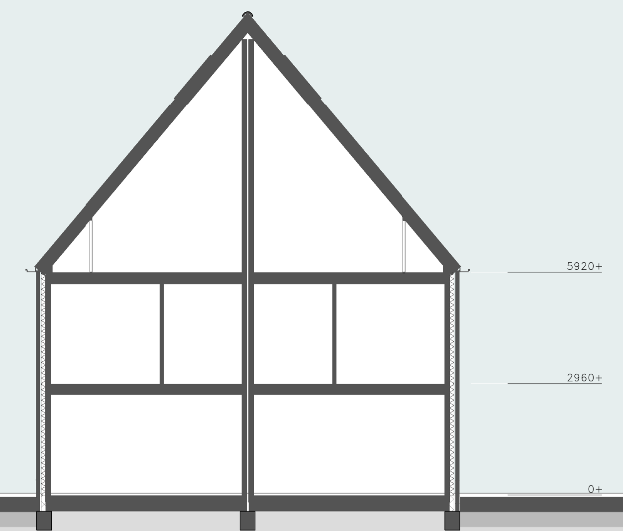
DOORSNEDE schaal 1 : 100
