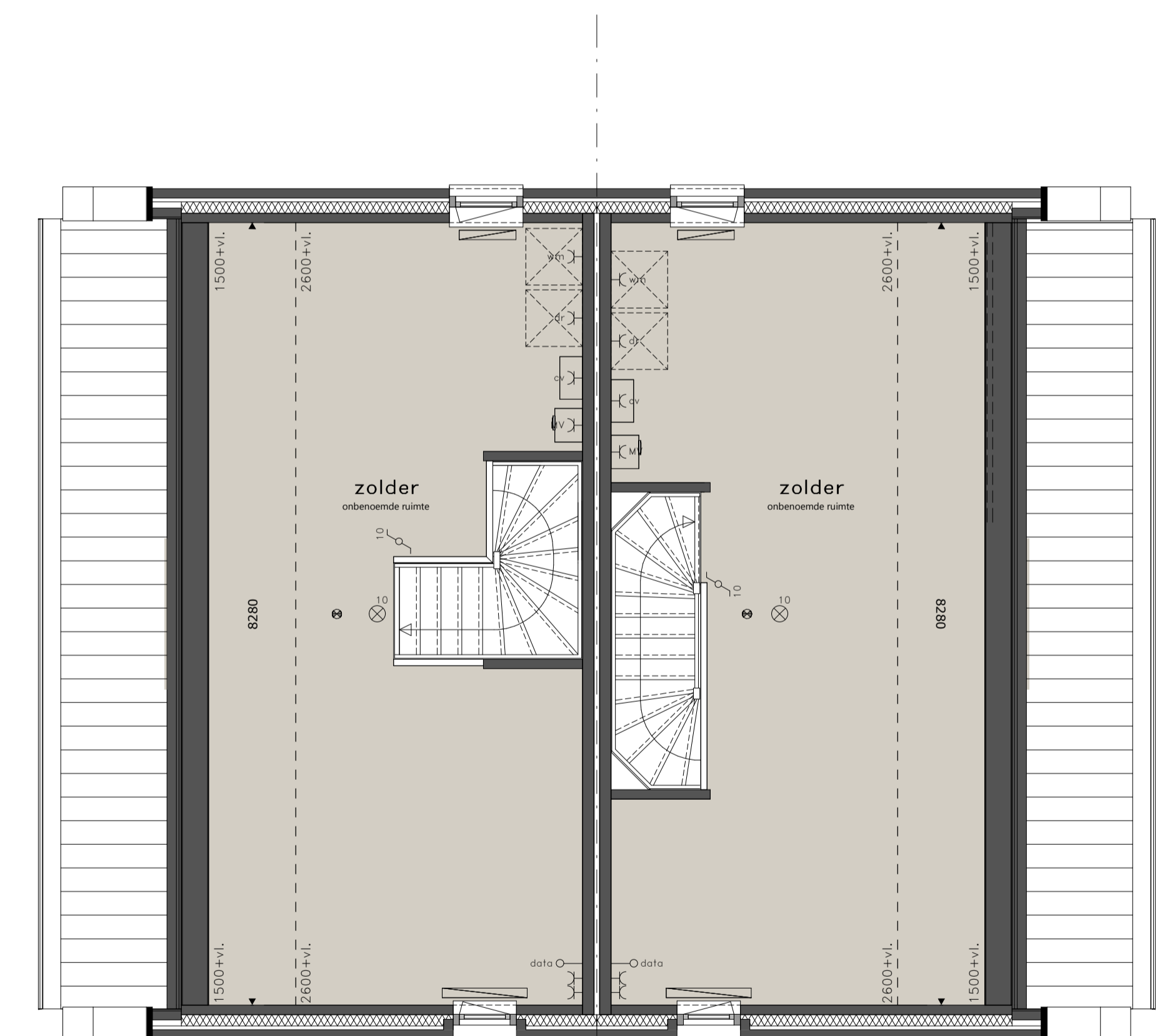
ZOLDER schaal 1 : 50
