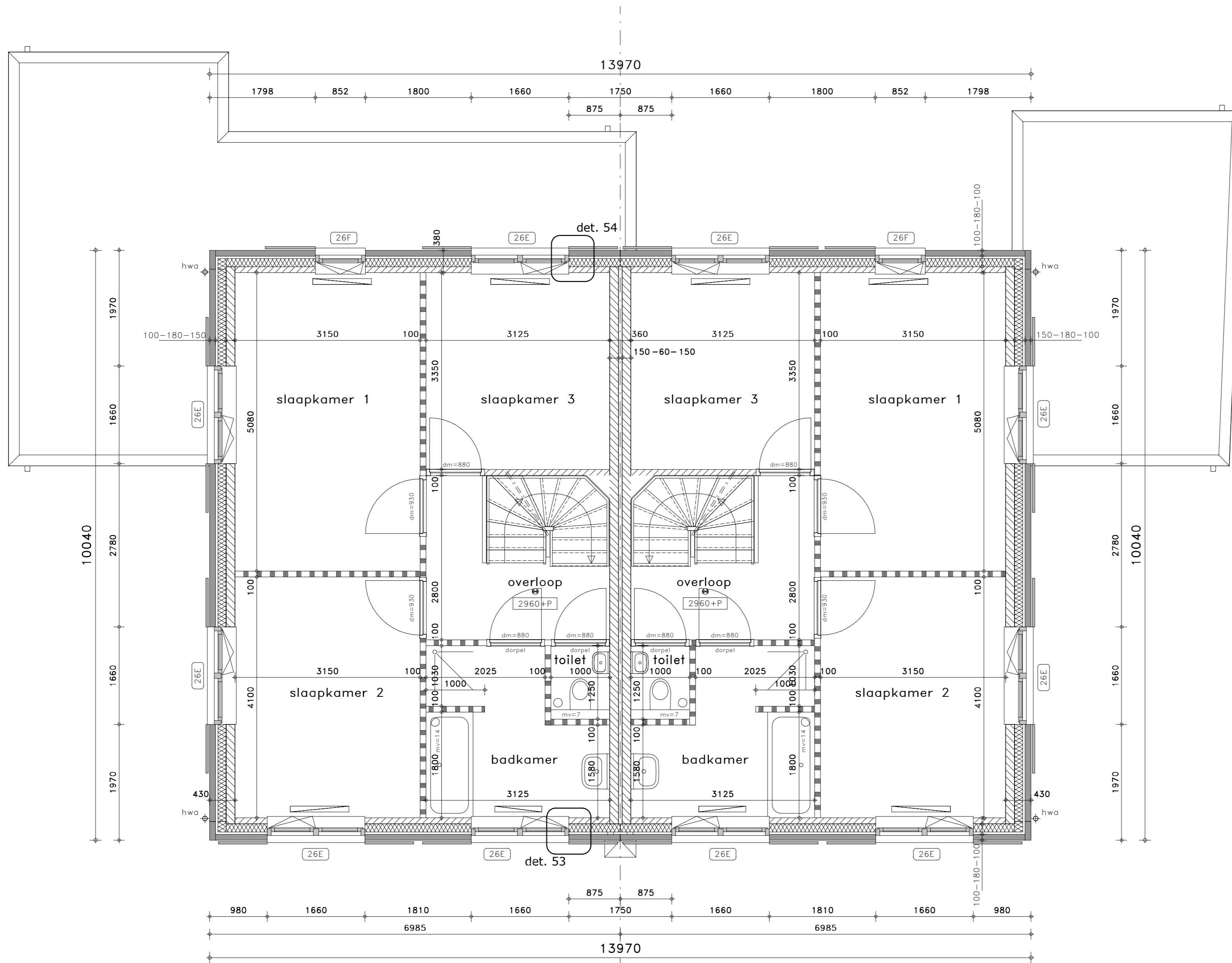
Blok 26 - 1e verdieping
